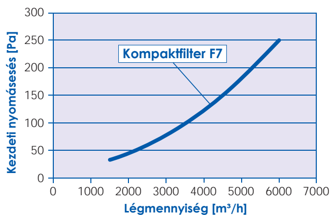
Kompaktszűrő diagramm F7
